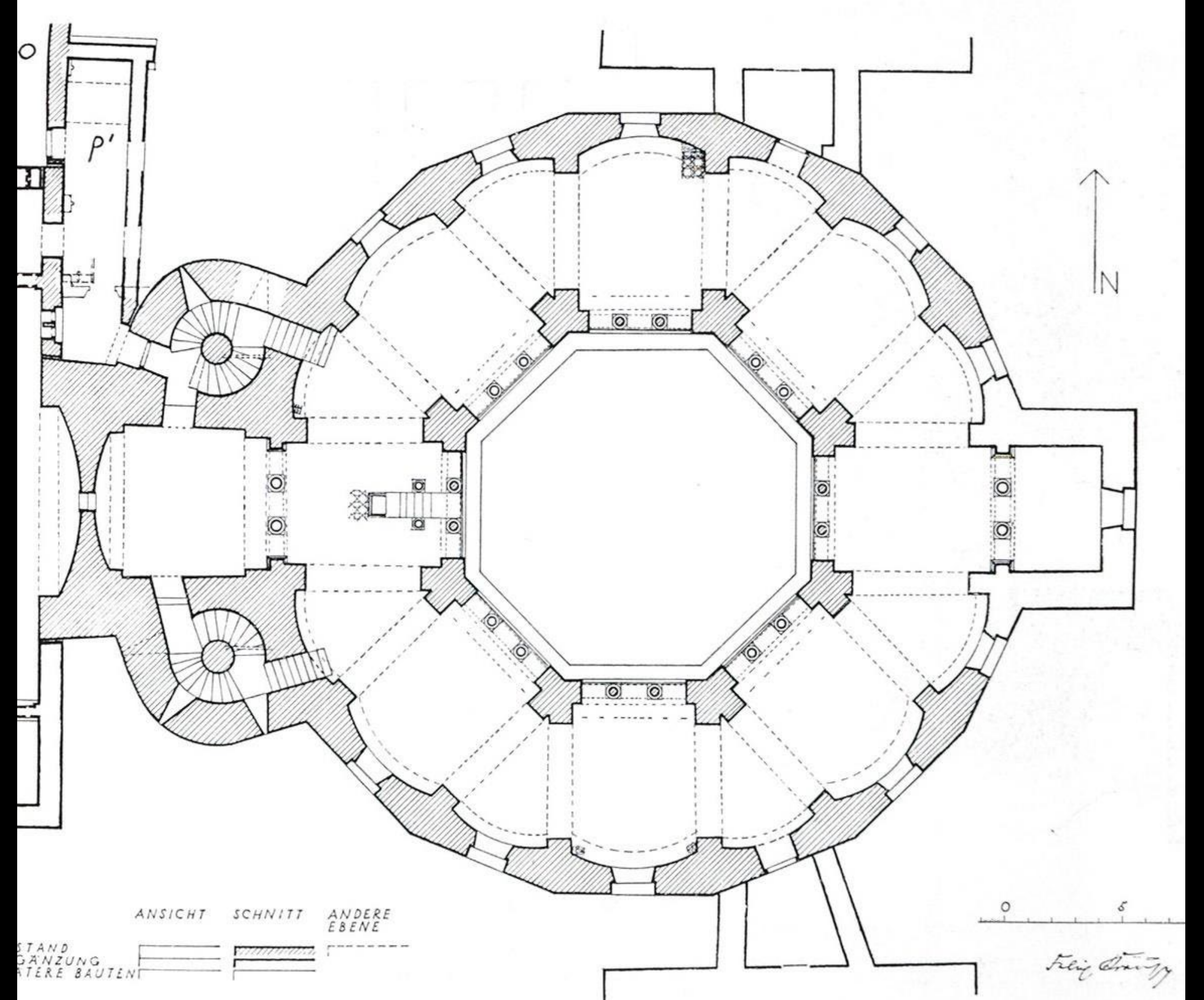
Niveau supérieur: voûte en berceau / Tonnegewölbe
