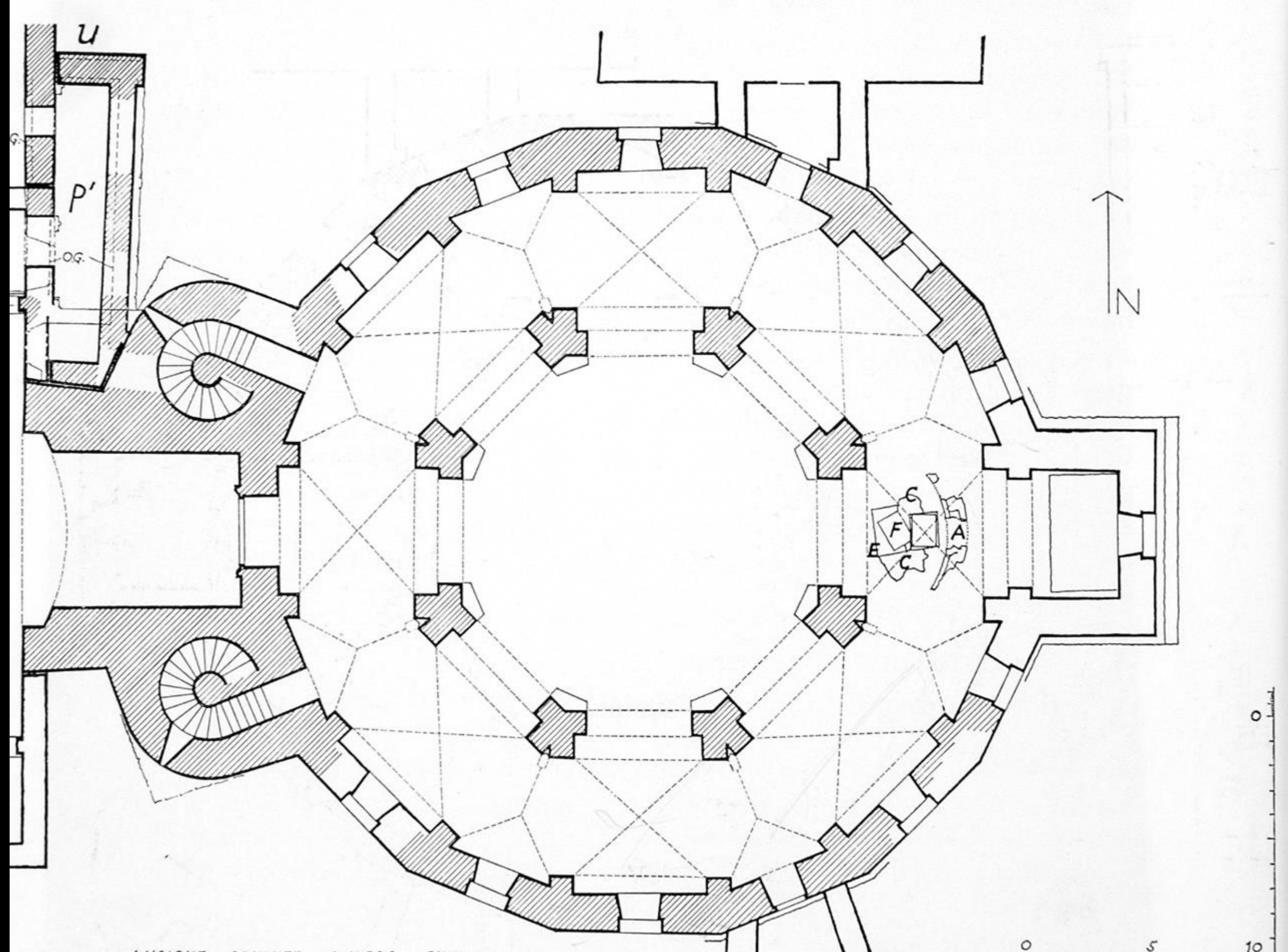
Niveau inférieur : voûte d'arêtes / Kreuzgratgewölbe
