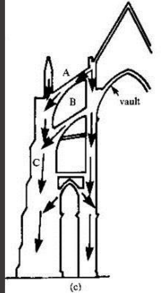
Strebewerk und Lastabtragung
