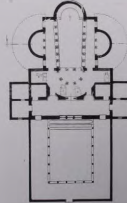
Τρίκλιτη Βασιλική (7ος αιώνας). Κάτοψη. Three-aisled basilica (7th century). Plan.
