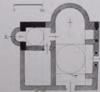
Μεγάλη Παναγιά (12ος αιώνας). Κάτοψη. Megali Panagia (12th century). Plan.
