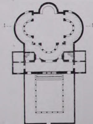
Τετράκογχος ναός (5ος αιώνας). Κάτοψη. Tetraconch church (5th century). Plan.
