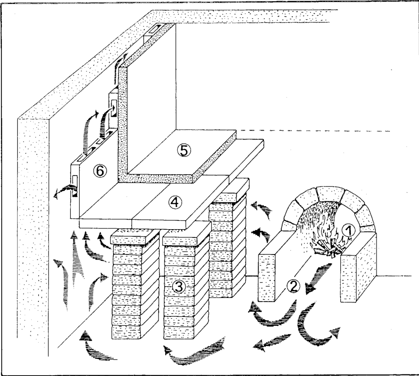
Hypocauste
