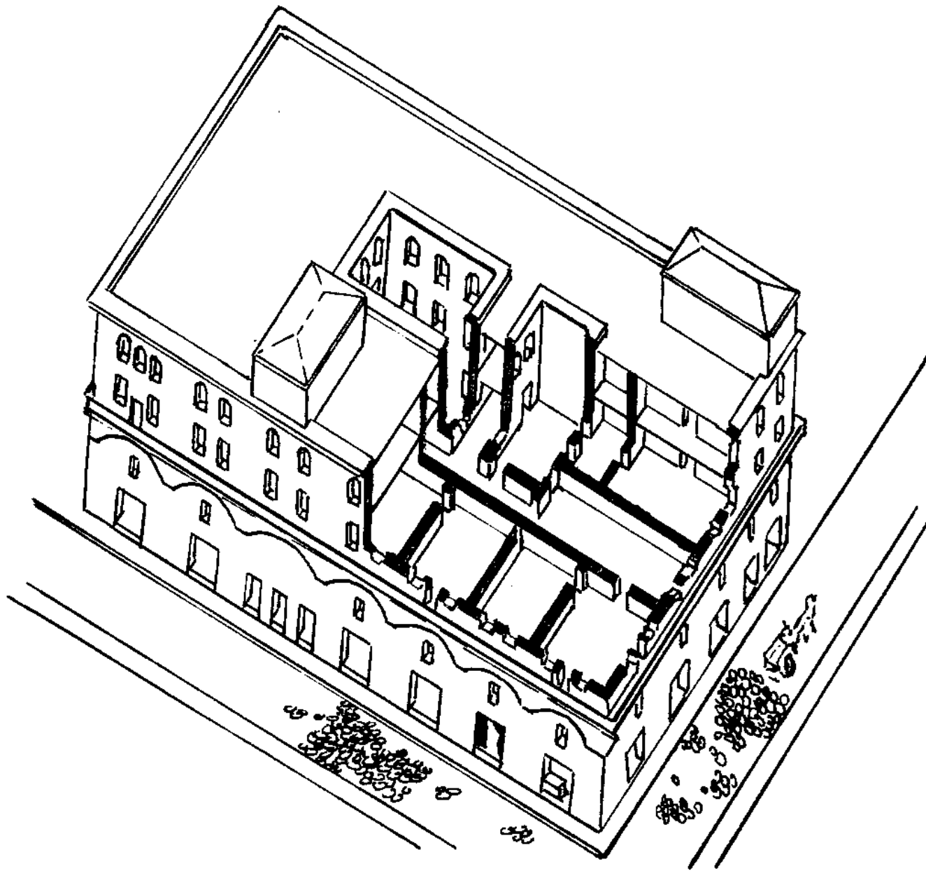
134. Immeuble d'Ostie. Coupe axonométrique
