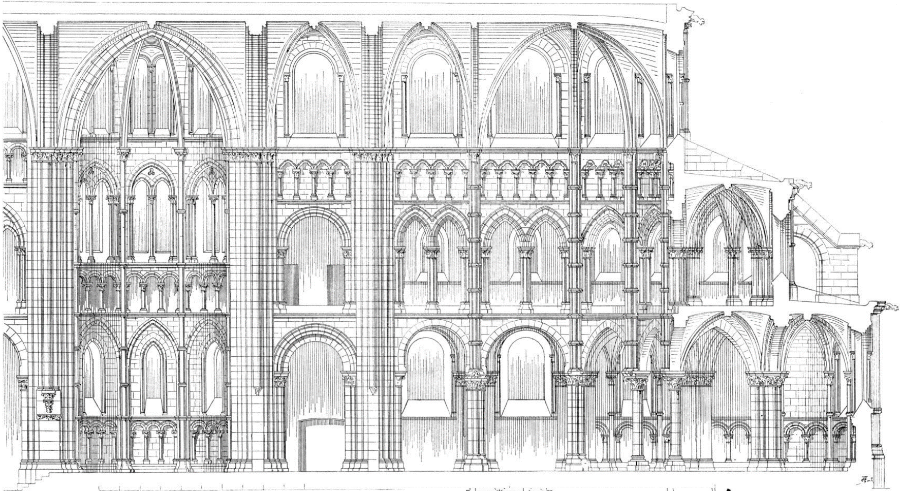
Noyon: Längsschnitt | coupe longitudinale
