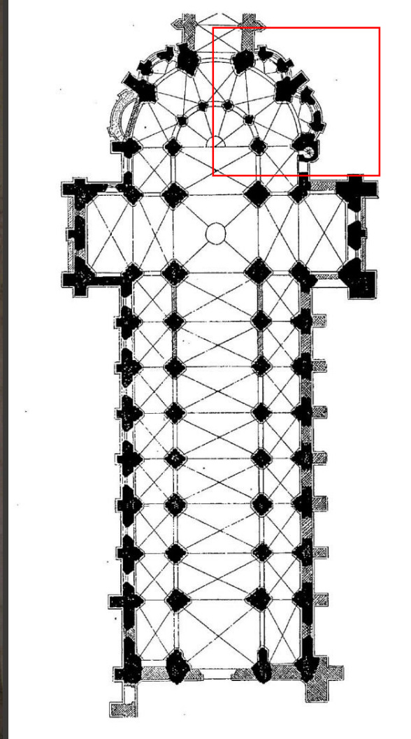
Allmähliche Auflösung der Wand in Fenster und Vorlagenbündel
