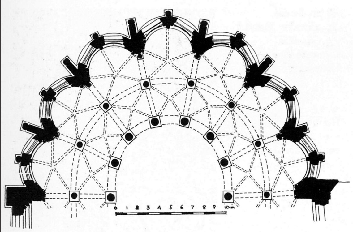
Saint Denis bei Paris – Ursprung der Gotik? Ab 1137 (Westbau) bzw. 1140 (Chor) umgebaut unter Abt Suger
