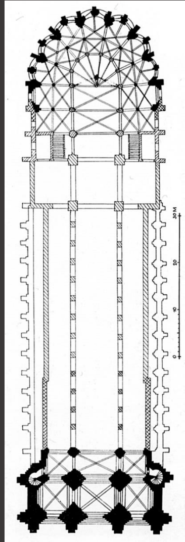
Westbau, erstes Bauprojekt unter Abt Suger An merowingisch-karolingische Kathedrale angefügt
